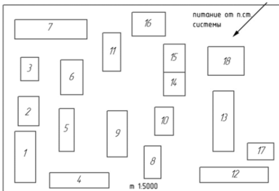
Рис. 1. 4. Генплан завода железобетонных изделий
